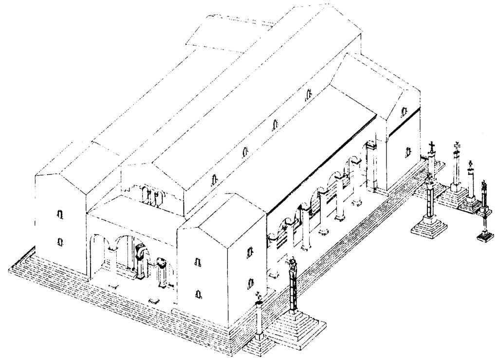
Նկ. 2. Երեւոյքի բազիլիկի վերակազմության փորձ: Հեղ. Պ.Տոնապետյան, կատարում՝ Դ.Ոլլիկյե (LA3M, 2012 թ.):
