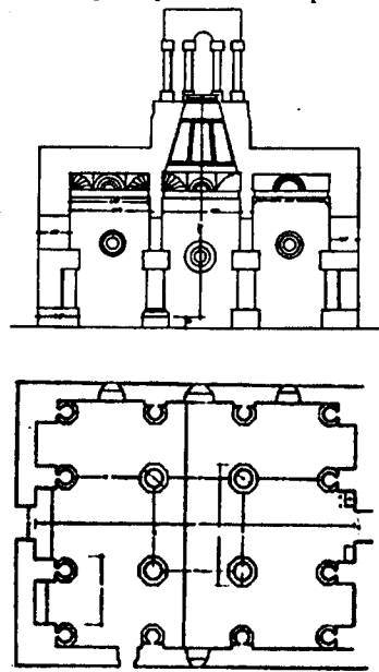
Рис. 1. Оромос, жаматун, план и продольный разрез по Торосу Тораманяну (Baladian et Thierry, Le couvent de Horomos , 2002)
